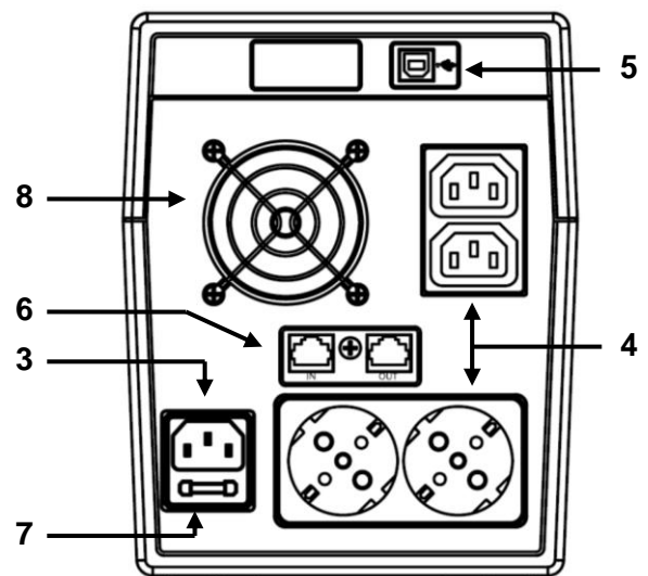
Vista posteriore UPS NemoLCD 200-300
