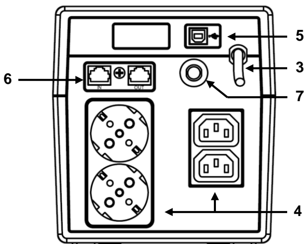
Vista posteriore UPS NemoLCD 160
